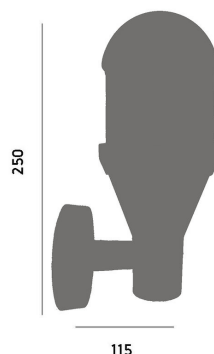
A189 Dimension : 115 x 108 x 250 mm. Material : Aluminium-Polycarbonate Color : Black
