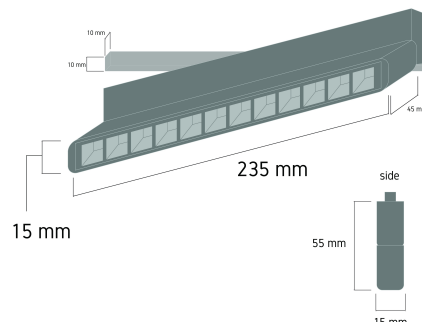
Mini MARCO P 12 3408019
