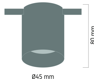
Mini Tube 6 3408039
